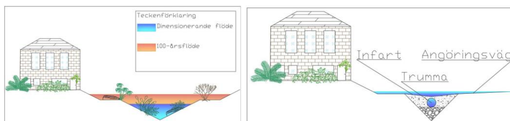
Bild 20 och 21: Principer för höjsättning för att skydda byggnader vid höga flöden med breddning kring diken (vänstra bilden) samt vid infarter (högra bilden). Bilder ur dagvattenutredningen, Ramboll.
