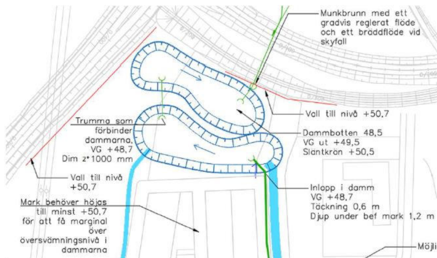
Figur 33. Föreslagna dagvattendammar längst i norr och markhöjder. (Ramböll, 2021).
