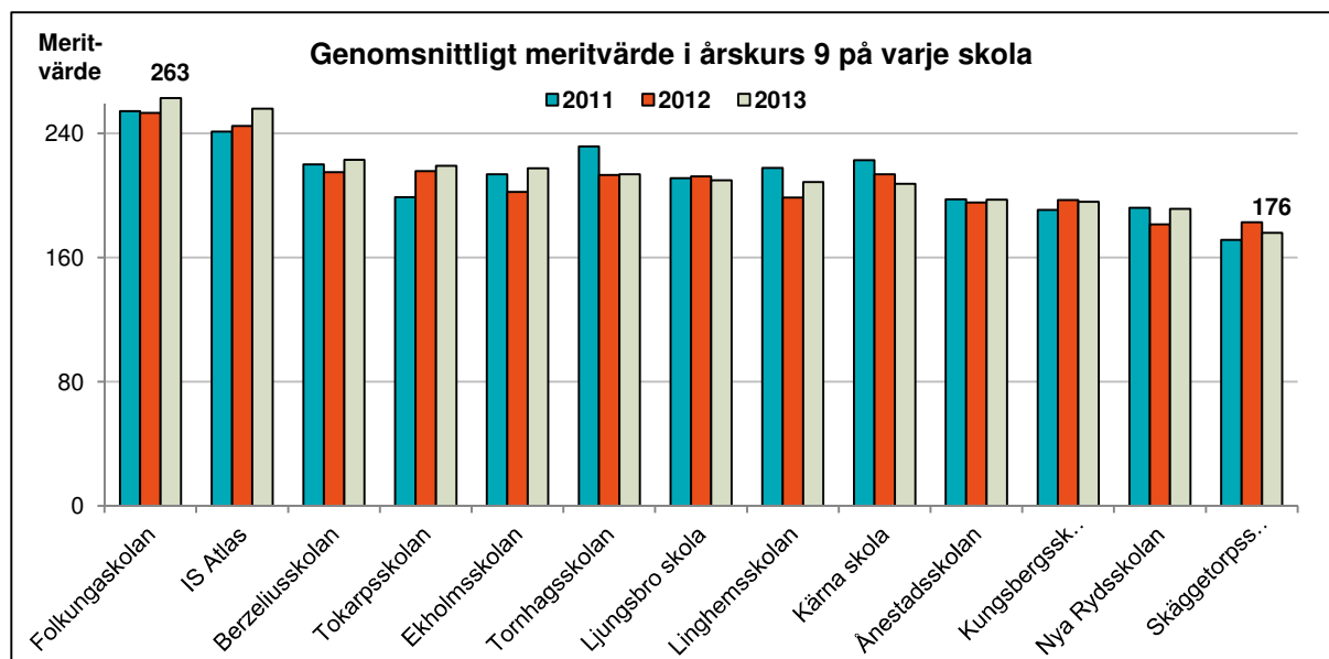
Diagram 3. Genomsnittligt meritvärde i årskurs 9 på varje kommunal skola i Linköping. Källa SCB.
