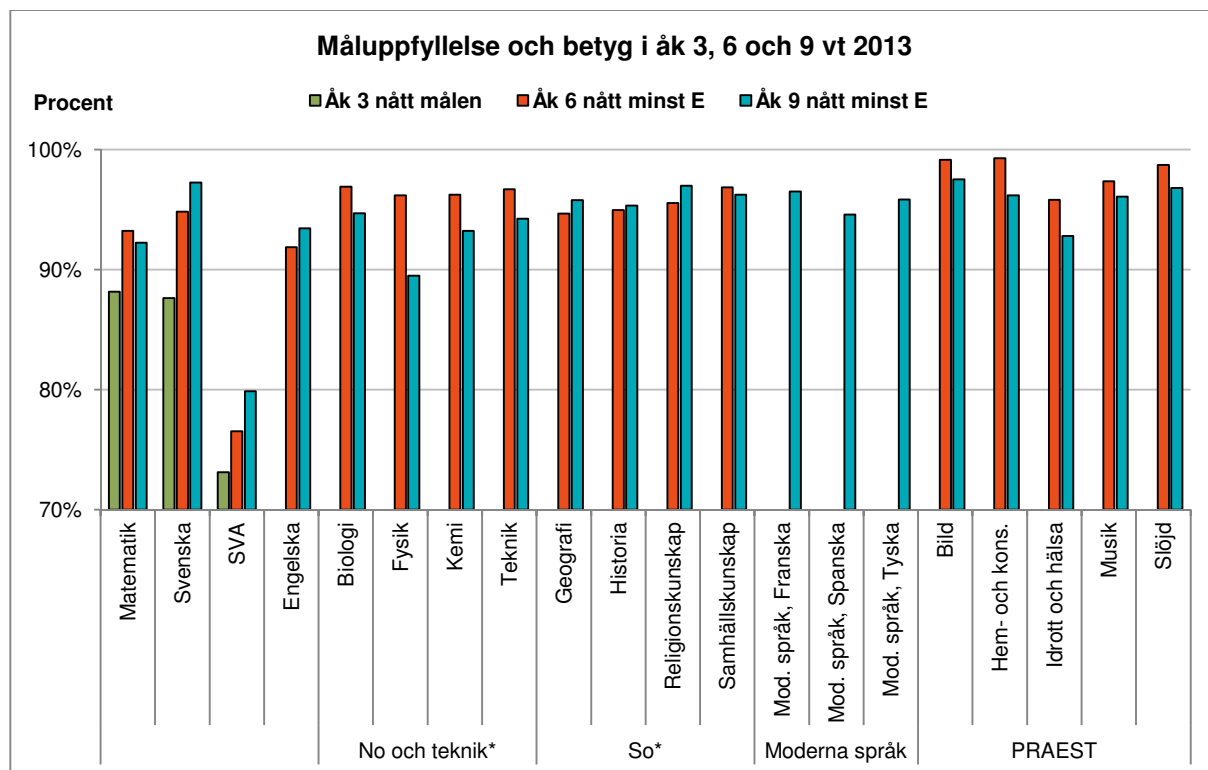
Diagram 1. Måluppfyllelse och betyg i årskurs 3, 6 och 9 2013. Källa SCB.
