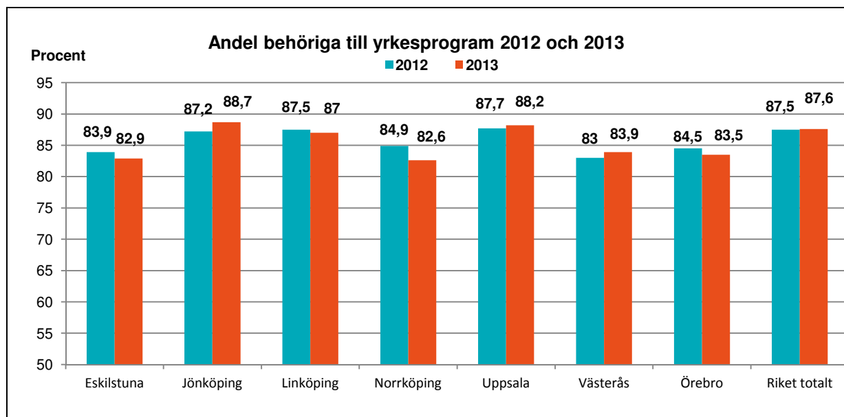
Diagram 2. Andel behöriga till yrkesprogram 2012 och 2013. Källa SCB.
