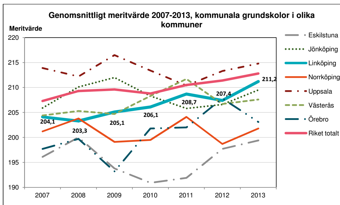
Diagram 4. Genomsnittligt meritvärde 2007-2013, kommunala grundskolor i olika kommuner. Källa SCB.
