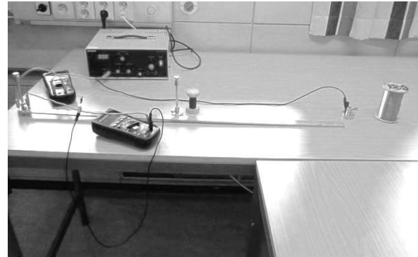
Bild 2. Försökstillställning.
